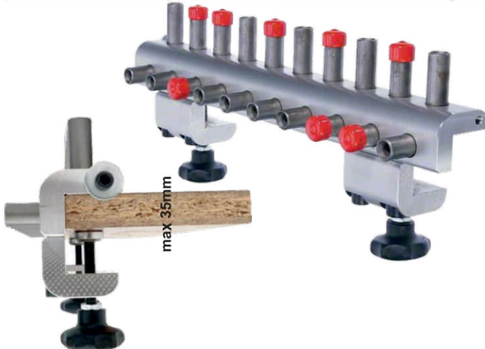
príklad vrtania do plochy príklad vrtania do hrany príklad vrtania do plochy
