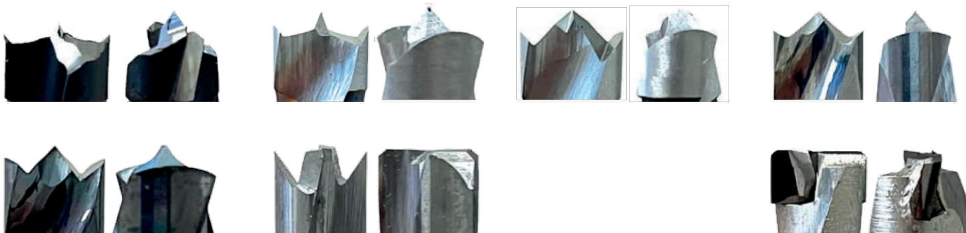
Druhy kolíkových vrtákov pre nepriebežné otvory
