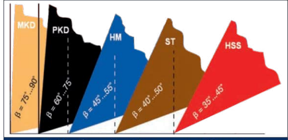
Závislosť rezného klinu na materiály ostria
