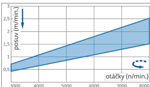
Závislosť otáčok a posuvu
