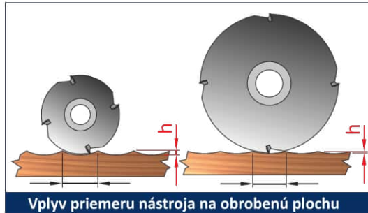
Vplyv priemeru nástroja na obrobenú plochu
