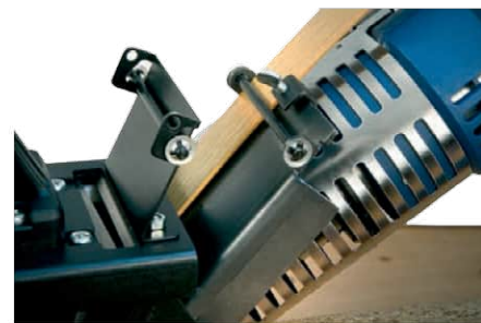
Teplovzdušná olepovačka pre ABS hrany 1mm s naneseným lepidlom.
