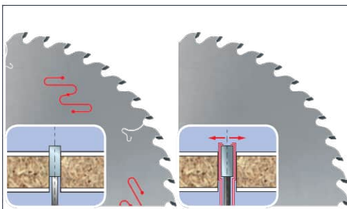
Antivibračné otvory v tele kotúča
