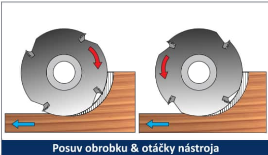
Posuv obrobnku & otáčky nástroja
